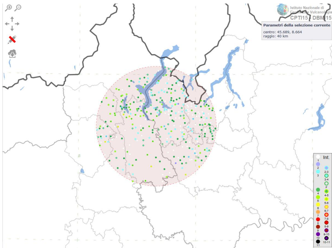
Figura 19: Carta rappresentativa degli eventi sismici nel periodo 1000-2014 nei dintorni di Cardano al Campo, distinti per intensità macrosismica
