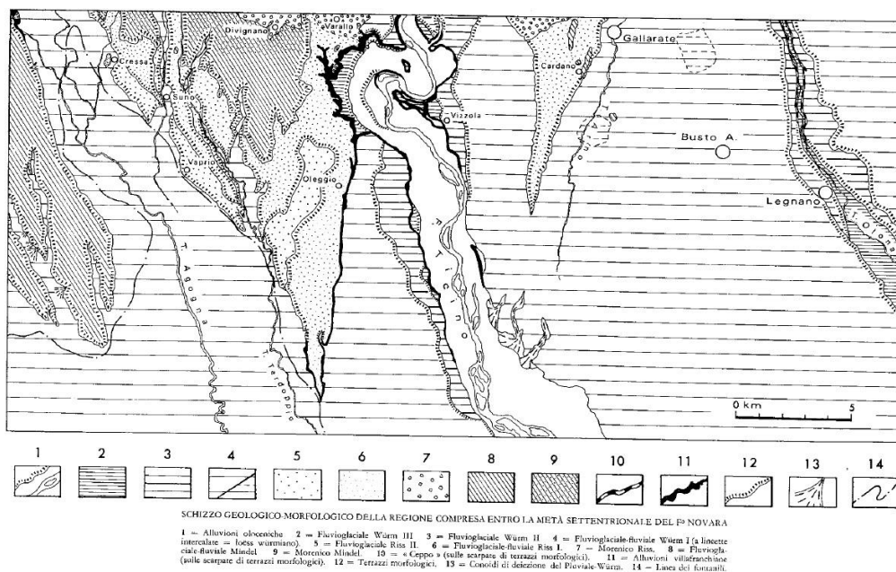
Figura 9: Schema geologico-morfologico della porzione settentrionale del Foglio Novara (Fonte: Note Illustrative Foglio Novara)
